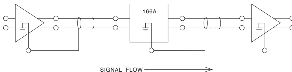
Abb. 4: Signalfluß (symmetrische Beschaltung)
